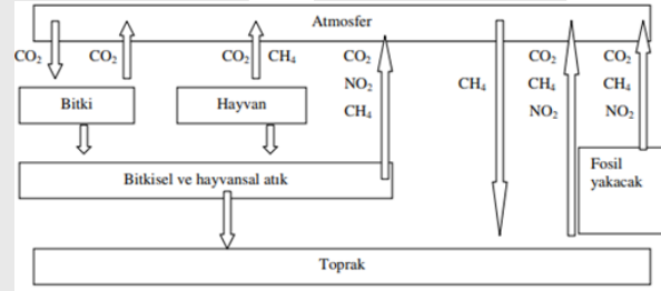
Şekil 1. Zirai Ekosisteme Bağlı Sera Gazlarının Kaynakları ve Depoları (H. Köknaroglu ve T. Akunal, 2010)
