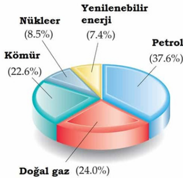
Şekil 1. Dünya genelinde kaynağına göre enerji kullanımı
